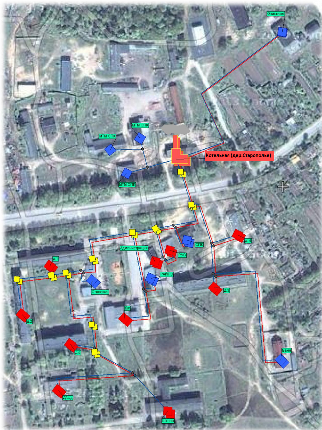
Рисунок 4. Схема горячего водоснабжения от котельной (дер. Старополье).
